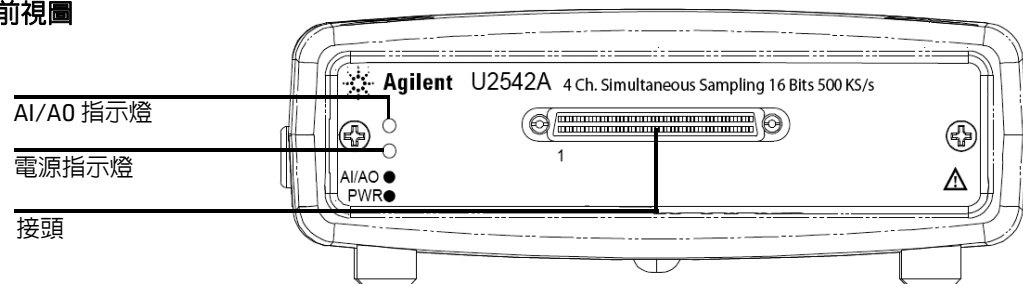
前視圖
