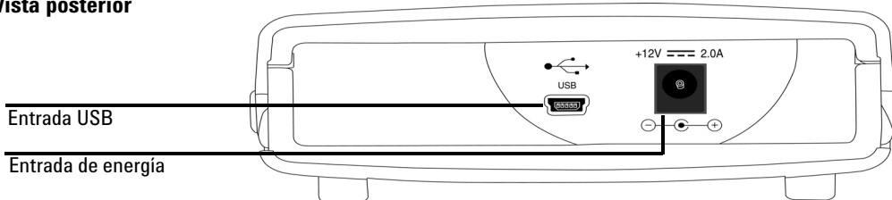
Vista posterior
